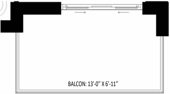
VARIANTES BALCON unités 206-208-308-310-408-410-508-510-608-610
